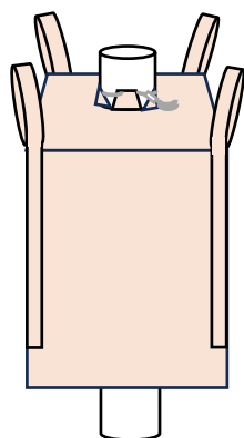
角型4本吊り投排口付きタイプ
