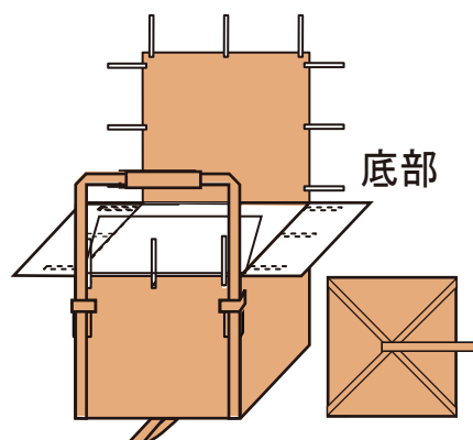
角型2本吊り反転ベルト付きタイプ
